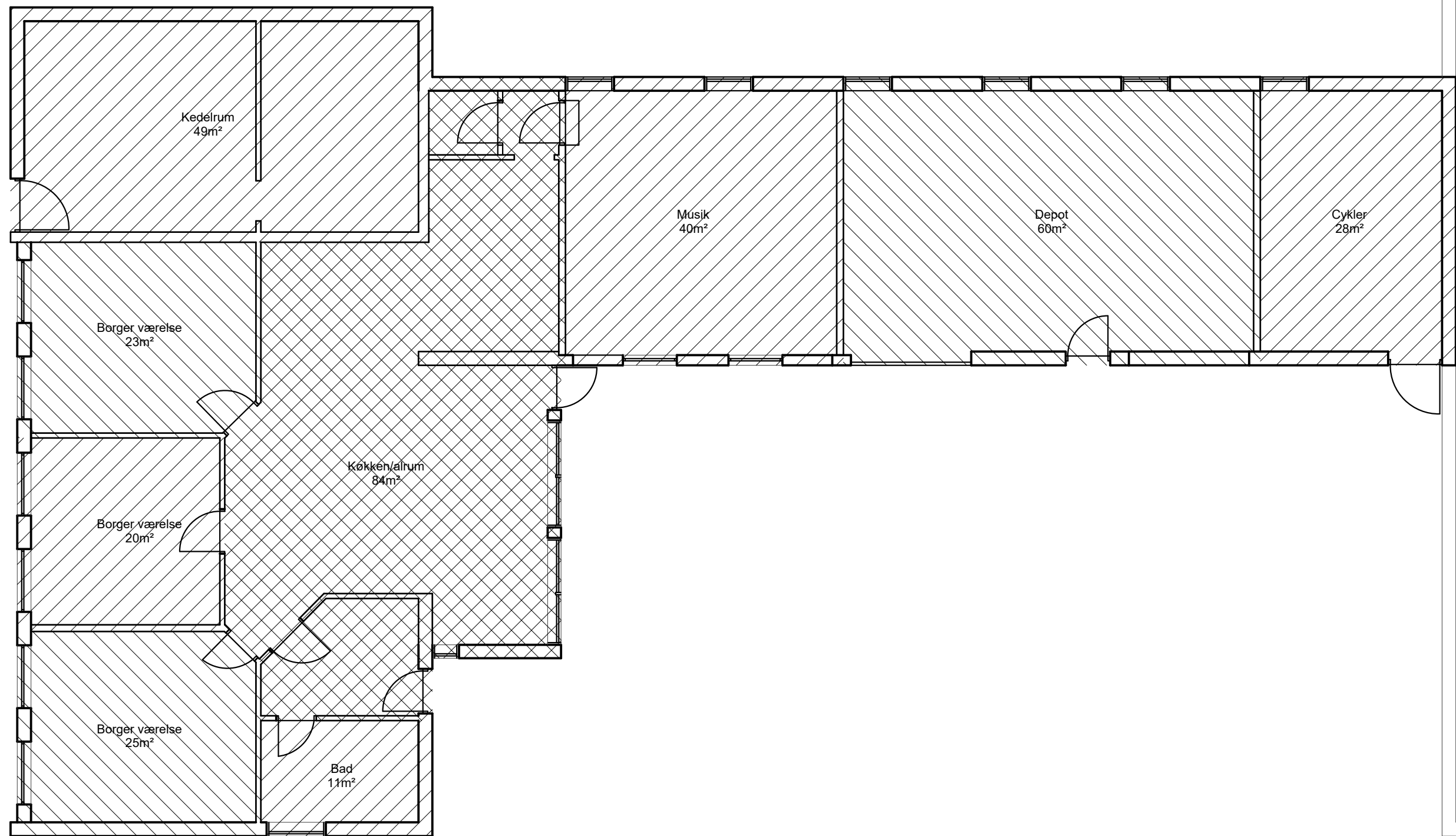
PLAN 1:100 BYGNING E, 342m 2 Arealer på diverse rum Hobro den 3. marts 2020
