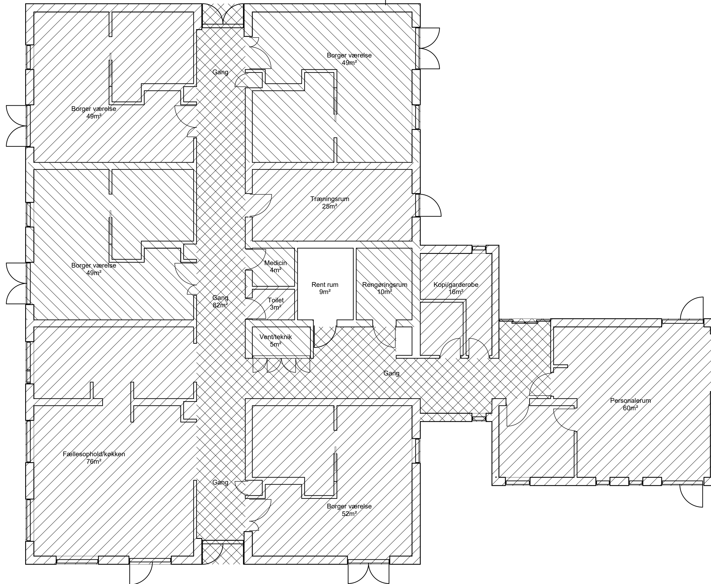
PLAN 1:100 BYGNING C, 490m 2 Arealer på diverse rum Hobro den 3. marts 2020
